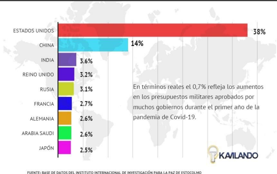
Gráfico 2: Mayor Gasto Militar Mundial
