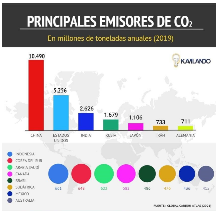
Gráfico 1: Principales emisores de CO2
