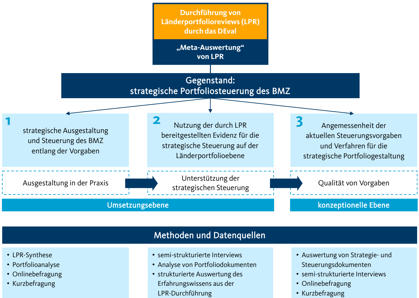
Abbildung 1 Überblick Evaluierungsdesign
