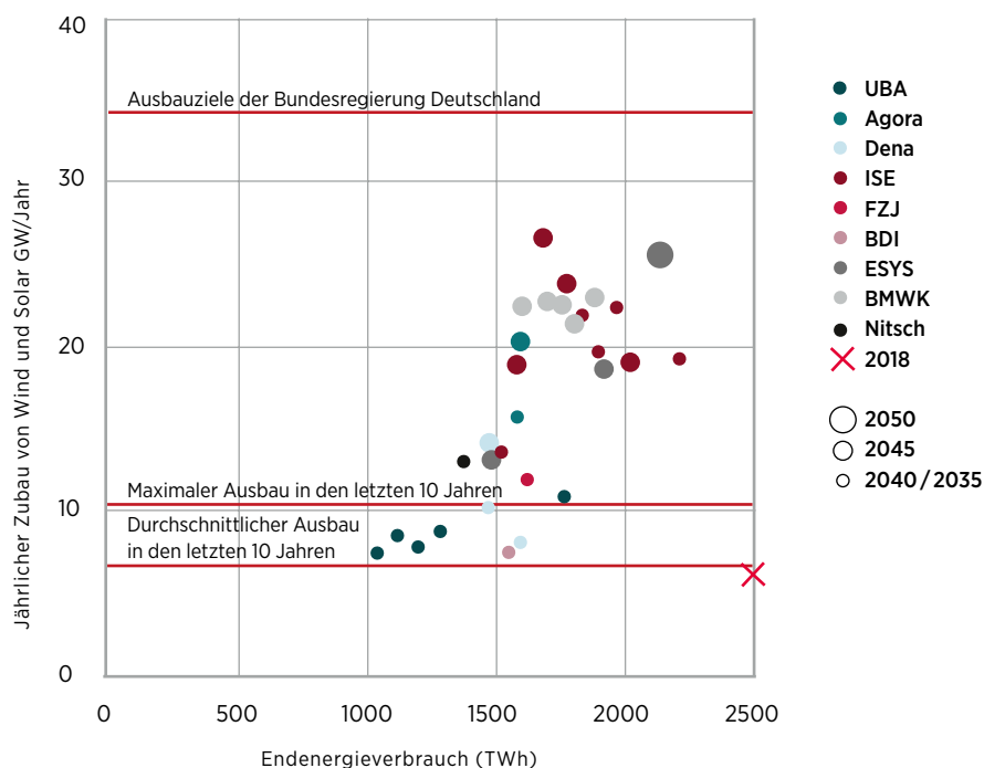
Endenergieverbrauch und jährlich installierte Kapazität von Wind und Solar in unterschiedlichen Klimaneutralitäts-Szenarien (-95% bis -100% THG-Emissionen ggü. 1990) für Deutschland: Jeder Punkt steht für ein Szenario, die Farben sind die Studien/ Autor*innen. Zum Vergleich sind der durchschnittliche Zubau der letzten zehn Jahre und der höchste erreichte jährliche Zubau angegeben.
