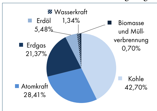
Grafik 1: Produktion von Primärenergieträgern (2006)
