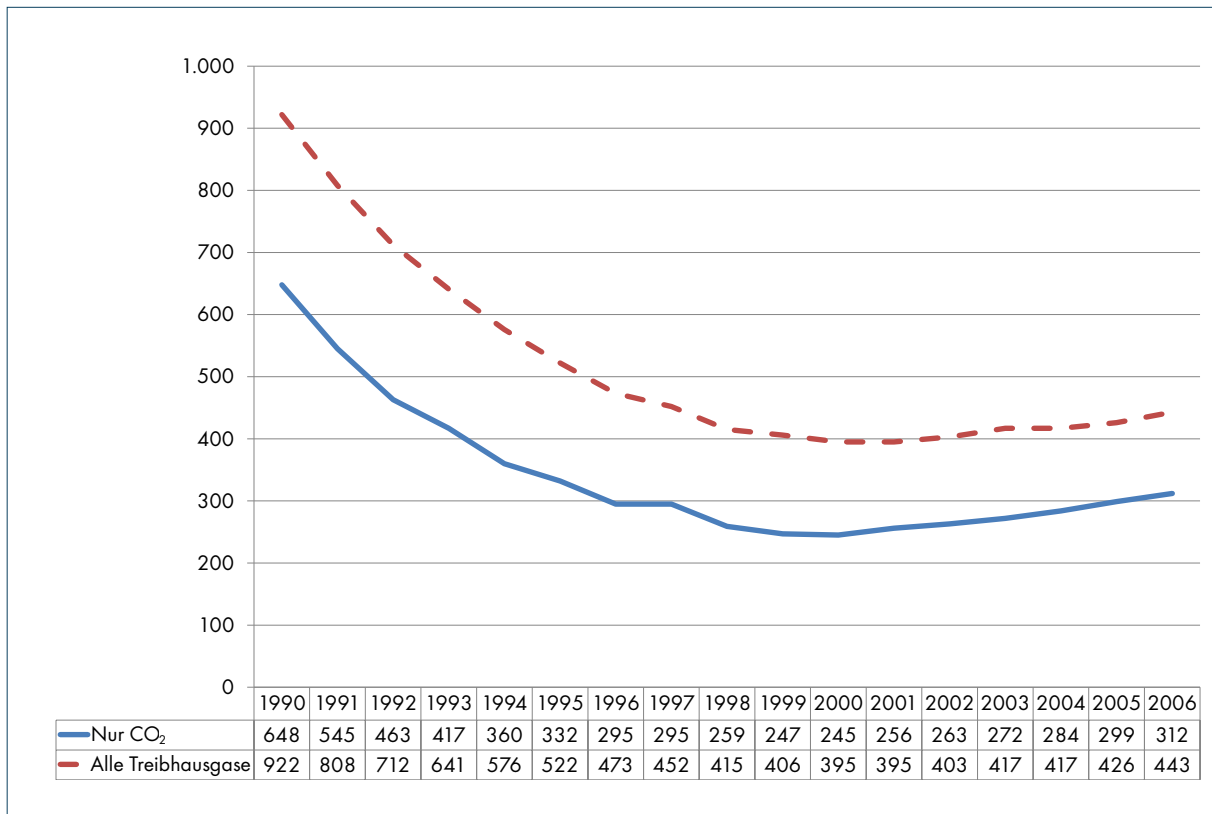
Grafik 5: Ukrainischer Ausstoß von Treibhausgasen 1990–2006 (CO 2 -Äquivalent in Mio. Tonnen)
