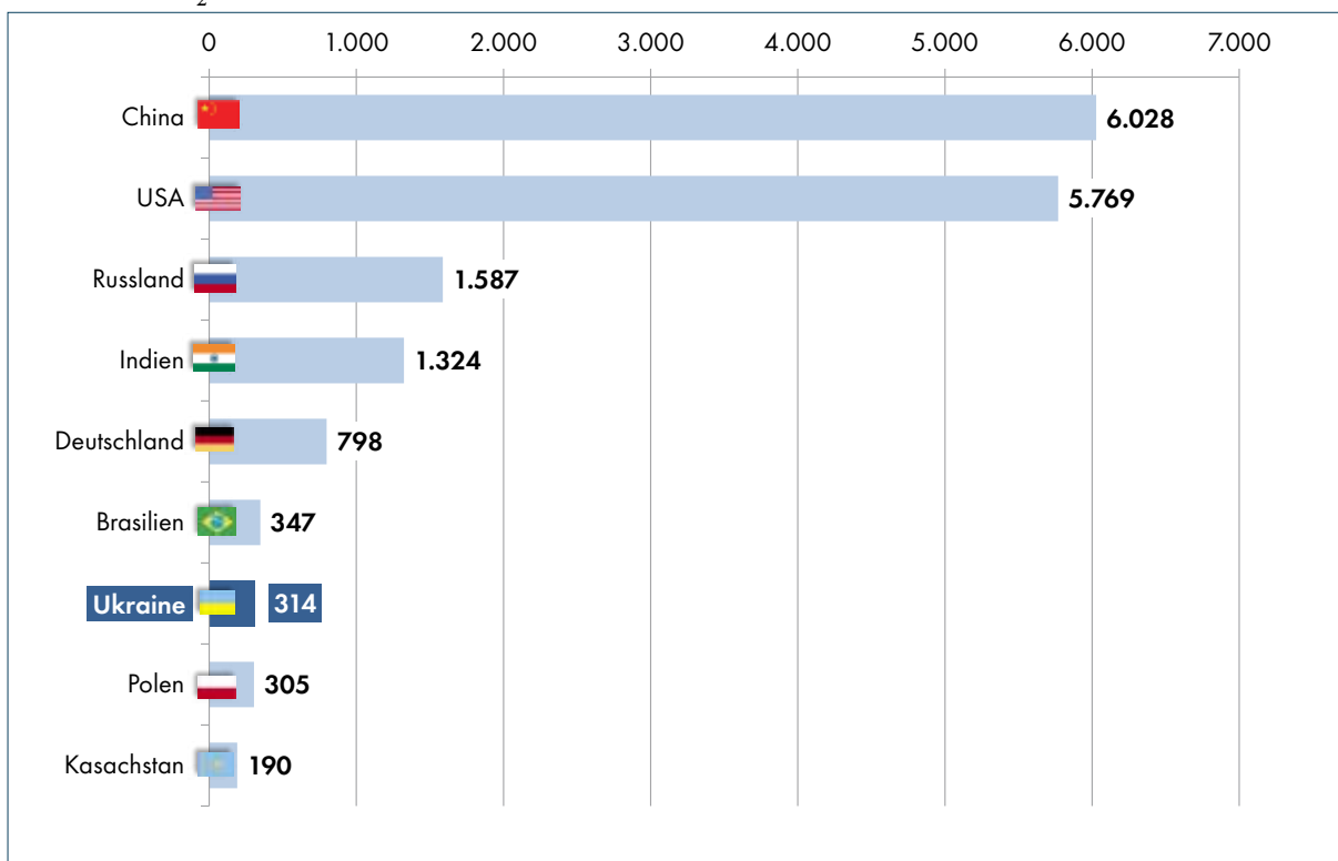
Grafik 2: CO 2 -Ausstoß in absoluten Zahlen (Mio. Tonnen, 2007)
