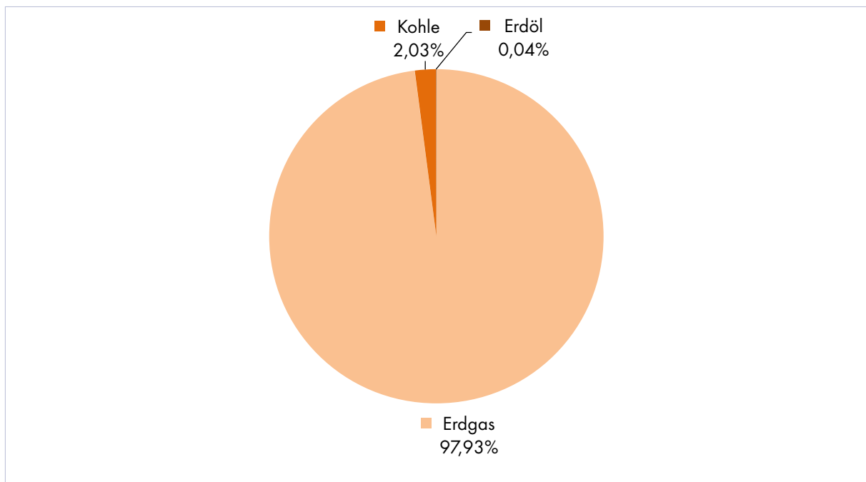
Grafik 3: Fernwärmeproduktion nach Energieträgern (2006)
