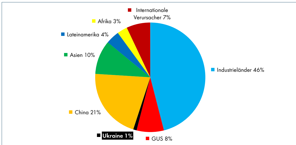
Grafik 1: Anteil am weltweiten CO 2 -Ausstoß (2007)
