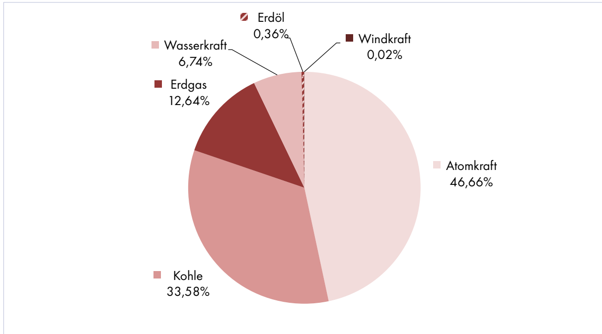
Grafik 2: Stromproduktion nach Energieträgern (2006)
