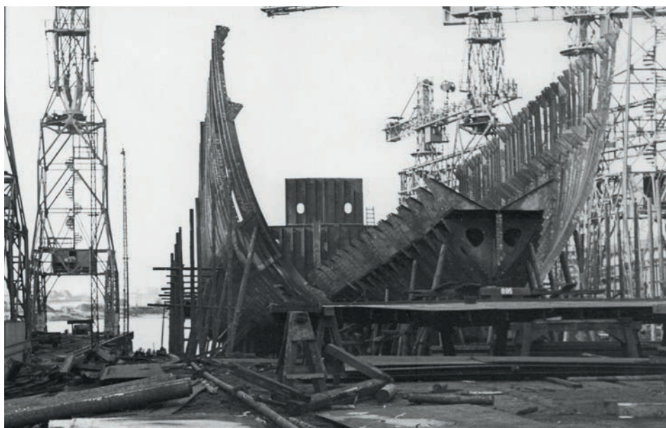
Abb. 13 Kombischiff GNEISENAU des NDL auf dem Helgen der AG »Weser«, 1935. (Foto: Hans Engelmeyer/Archiv DSM)
