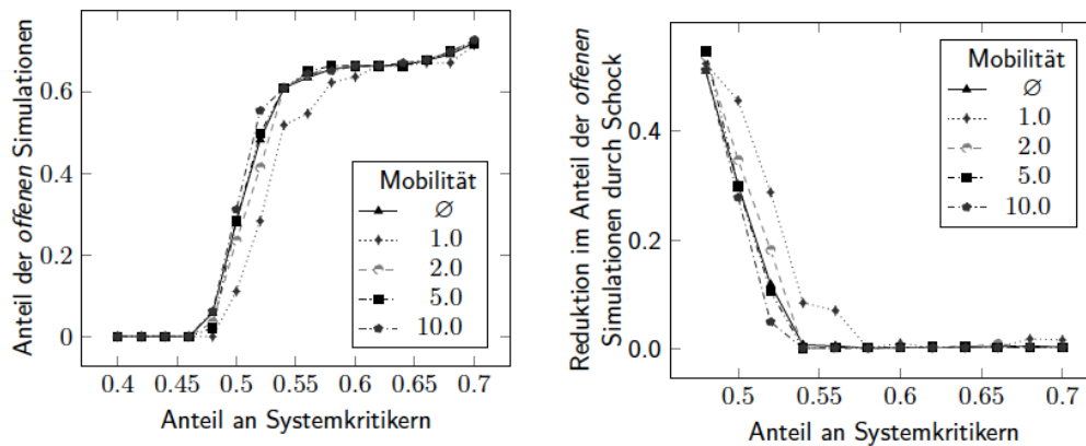
Abb. 7: Einfluss von Schocks in Runde 200 auf Simulationsergebnisse. Linke Seite: Anteil der offenen Simulationen nach einem negativen Schock, in Abhängigkeit vom Anteil der Systemkritiker. Rechte Seite: Differenz im Anteil der offenen Simulation mit und ohne Schock (vgl. Abb. 3)
