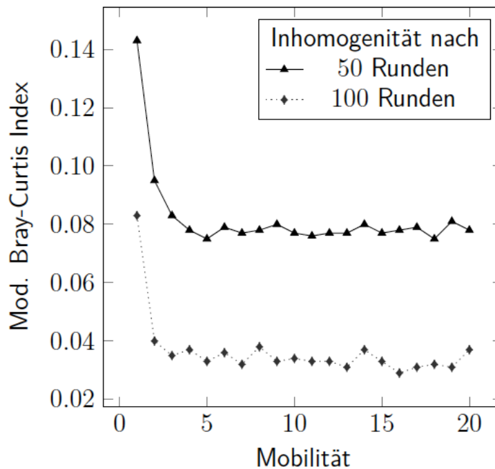
Abb. 4: Inhomogenität, gemessen im modifizierten Bray-Curtis Index nach 50 und 100 Runden, in Abhängigkeit von der Mobilität
