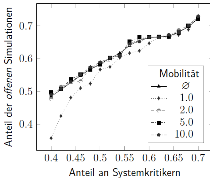
Abb. 3: Einfluss des Anteils der systemkritischen Akteure auf Anteil der offenen Simulationen für ausgewählte Mobilitätswerte.
