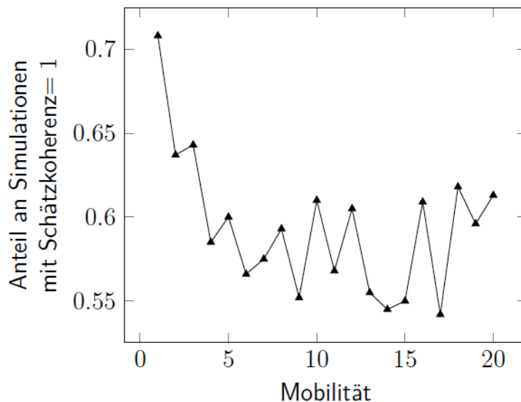
Abb. 6: Schätzkohärenz (Anteil der Simulationen, in denen regimekritische Akteure das Wechselklima höher wahrnehmen als regimetreue Akteure) in Abhängigkeit von der Mobilität
