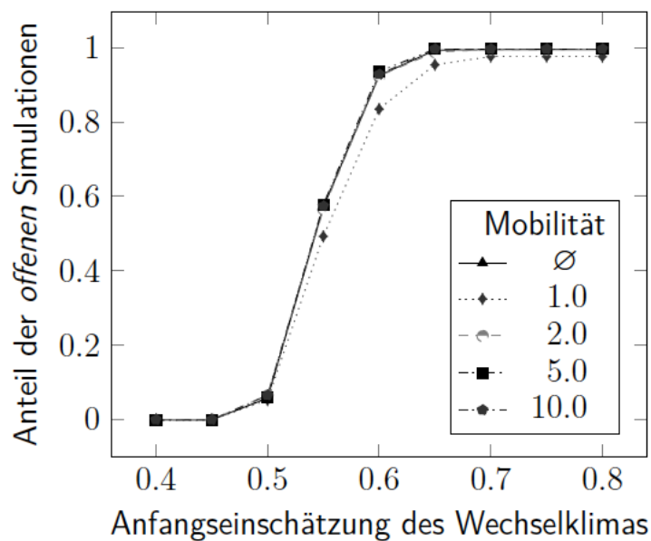
Abb. 2: Einfluss der Anfangseinschätzung des Wechselklimas auf Anteil der offenen Simulationen für ausgewählte Mobilitätswerte.
