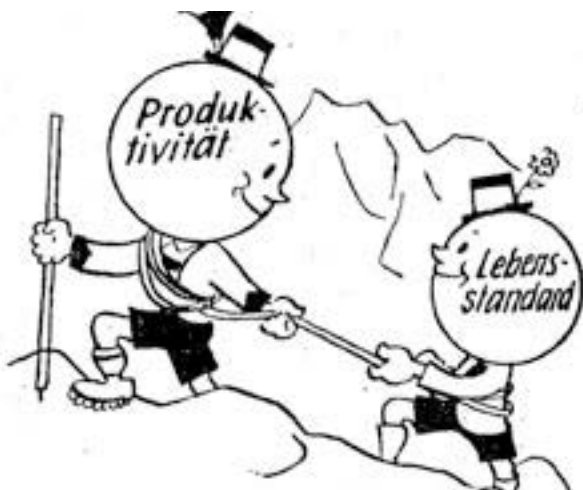
Abbildung 108: Produktivität, 1952
