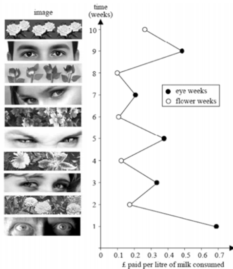
Abbildung 1: Der Observer-Effekt
