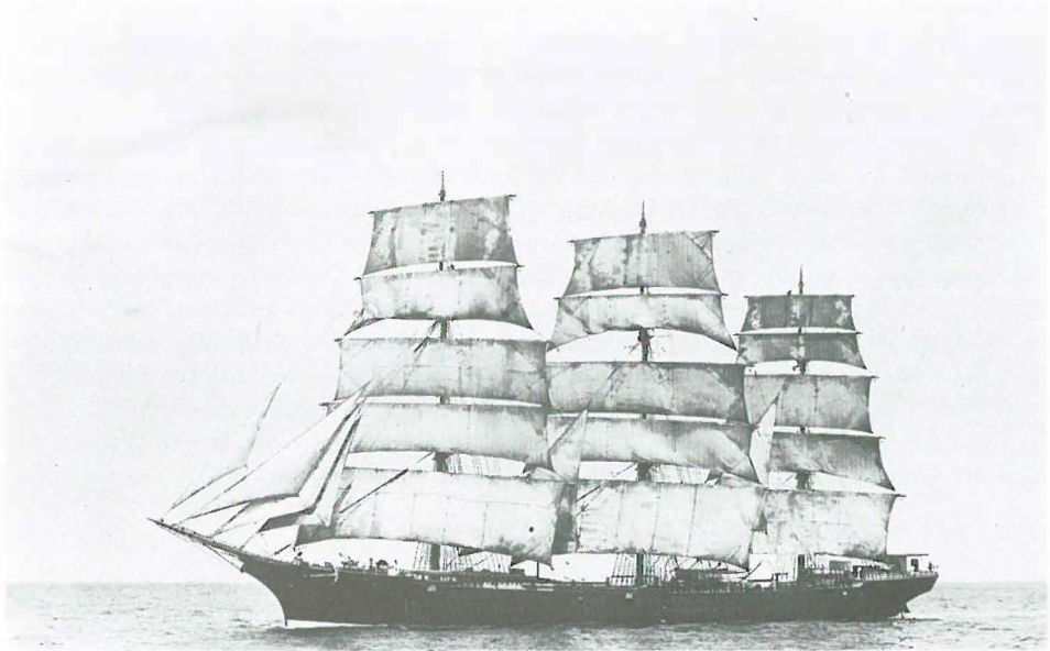
Das Vollschiff LASBEK, 1910 von England gekauft, machte bis 1914 drei Reisen nach Santa Rosalia. (Foto: Slg. Harold D. Huycke)
