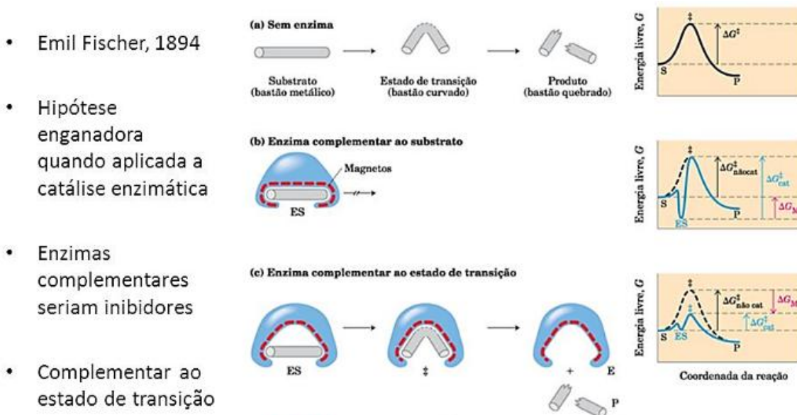
FIGURA 6-5 Uma enzima imaginária (bastonase) que catalisa a quebra de um bastão metálico.
