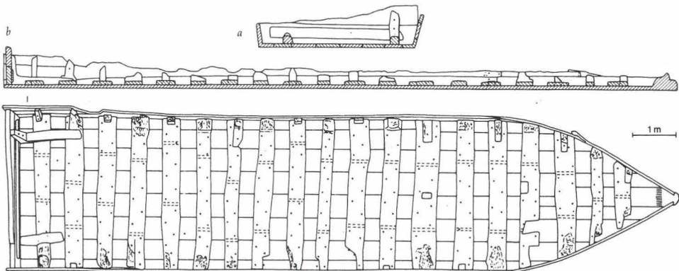
Abb. 15 Falsterbo, Schonen. Prahm zum Leichtern großer Seeschiffe (vor 1318).
