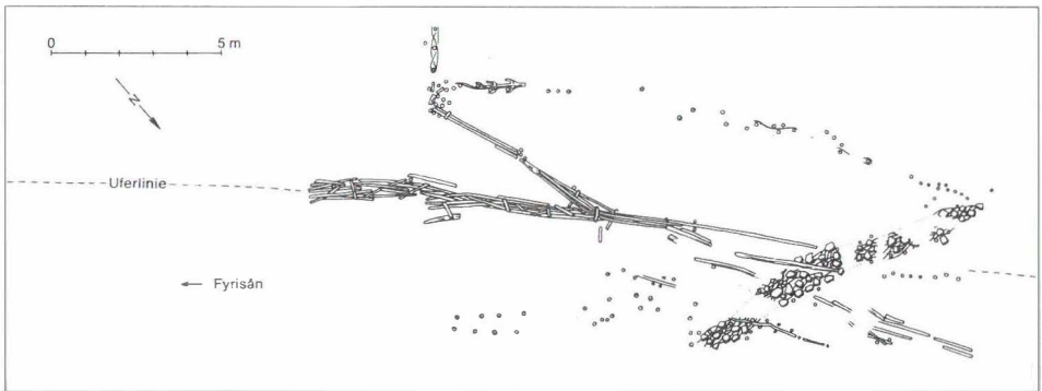
Abb. 16 Uppsala, Studentenholmen. Schiffslände mit Steinpflaster unter Wasser (etwa 11. Jahrhundert).
