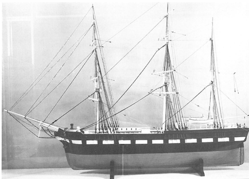
Der Bremer Auswanderersegler EDMUND (Ausstellung DSM, Foto: Marburg)
