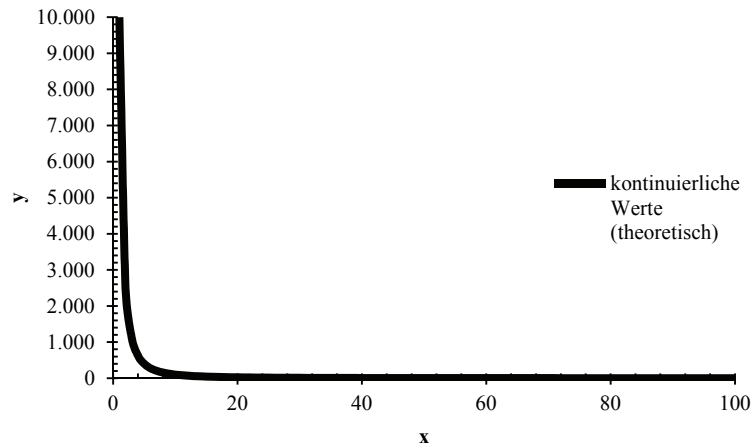
Abb. 1: Plot derselben Power-Law-Funktion mit den Werten c = 10.000 und \alpha = 2 .
