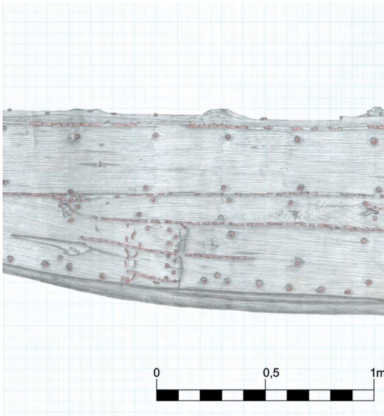
Abb. 24 Feldzeichnung des Unterbords auf der Backbordseite, Kalfatering, »Nachennaht« und Plankenverbindungen mit Butte und Schäftung. (Zeichnung: E. Augustin, archaeologie.de )
