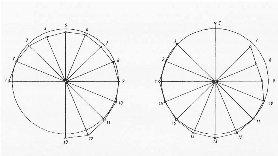
Abb. 3 Systematik des Pergamentverzuges (die Abweichungen wurden um den Faktor 10 überhöht dargestellt)
