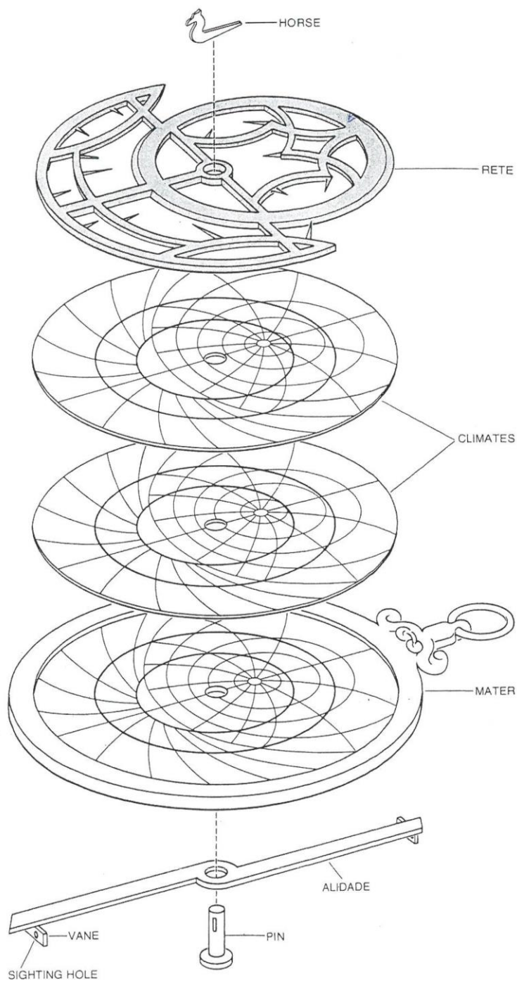
Abb. 2: Explosionsansicht eines Astrolabiums.
