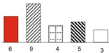
Häufigkeitsverteilung
