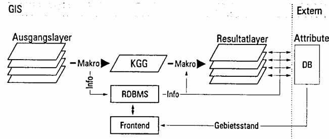
Abb. 11: Abbildung eines objektorientierten logischen Datenmodell mit Hilfe eines layerorientierten GIS und relationalen DBMS
